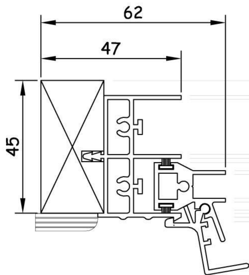
Horizontal Slider Jamb detail.
